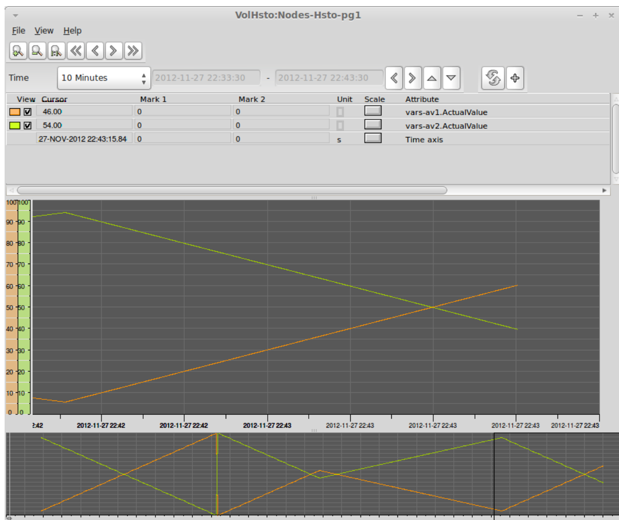
FIGURE 5 – Mode run sous Xtt : Historisation de variables
